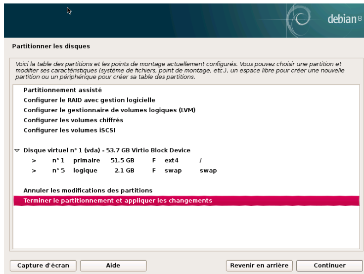
FIGURE 4.10 Valider le partitionnement
