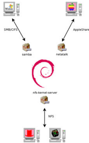
FIGURE 3.1 Cohabitation de Debian avec OS X, Windows et les systèmes Unix
